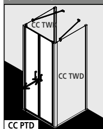
U-Kabina: CC PTD a CC TWD a CC TWD (strana 320) a 2x ZDSS VSS CC120 (strana 340)
